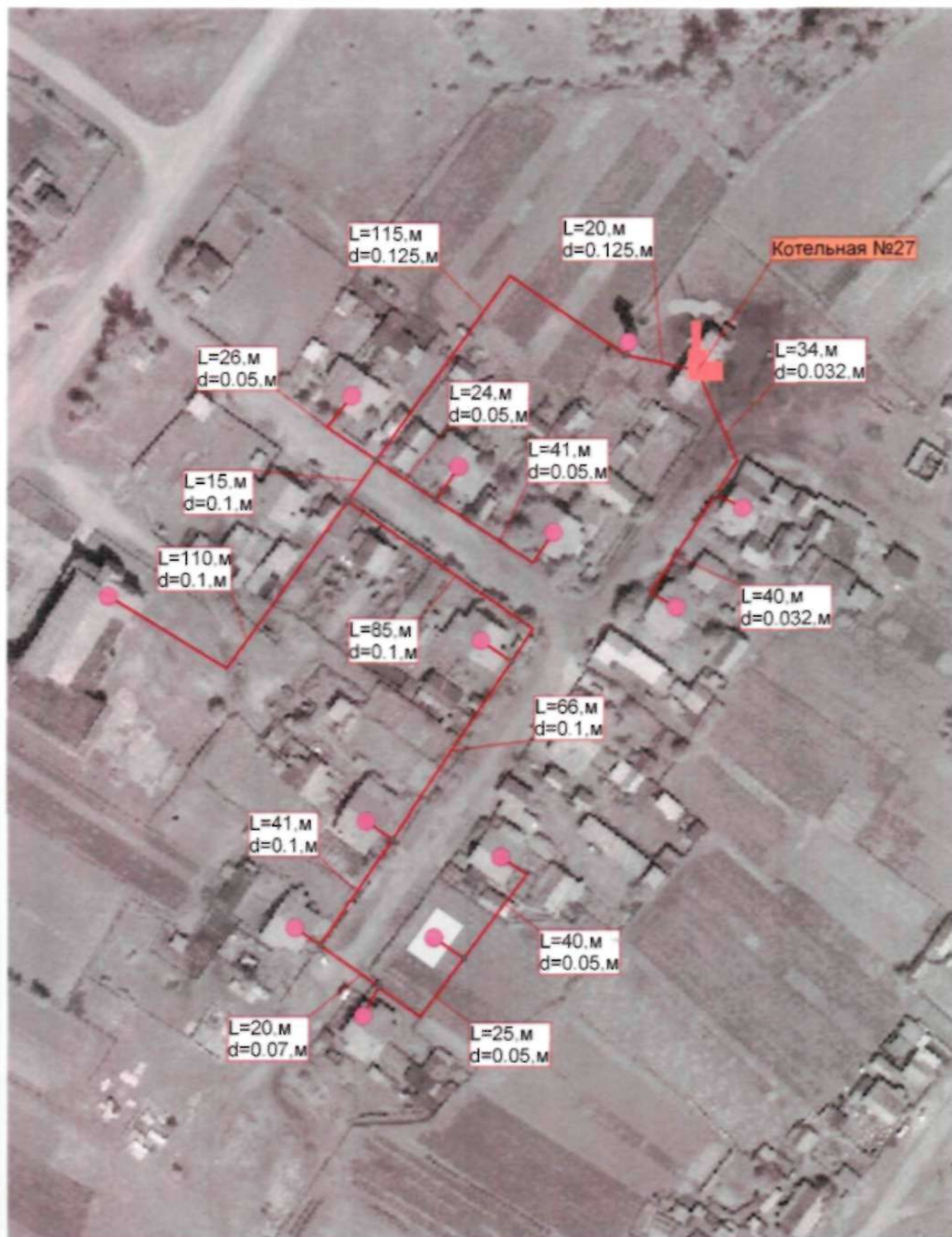
Рис. 2.5 – Схема теплоснабжения муниципального образования "Климоуцевский сельсовет" от котельной №27
