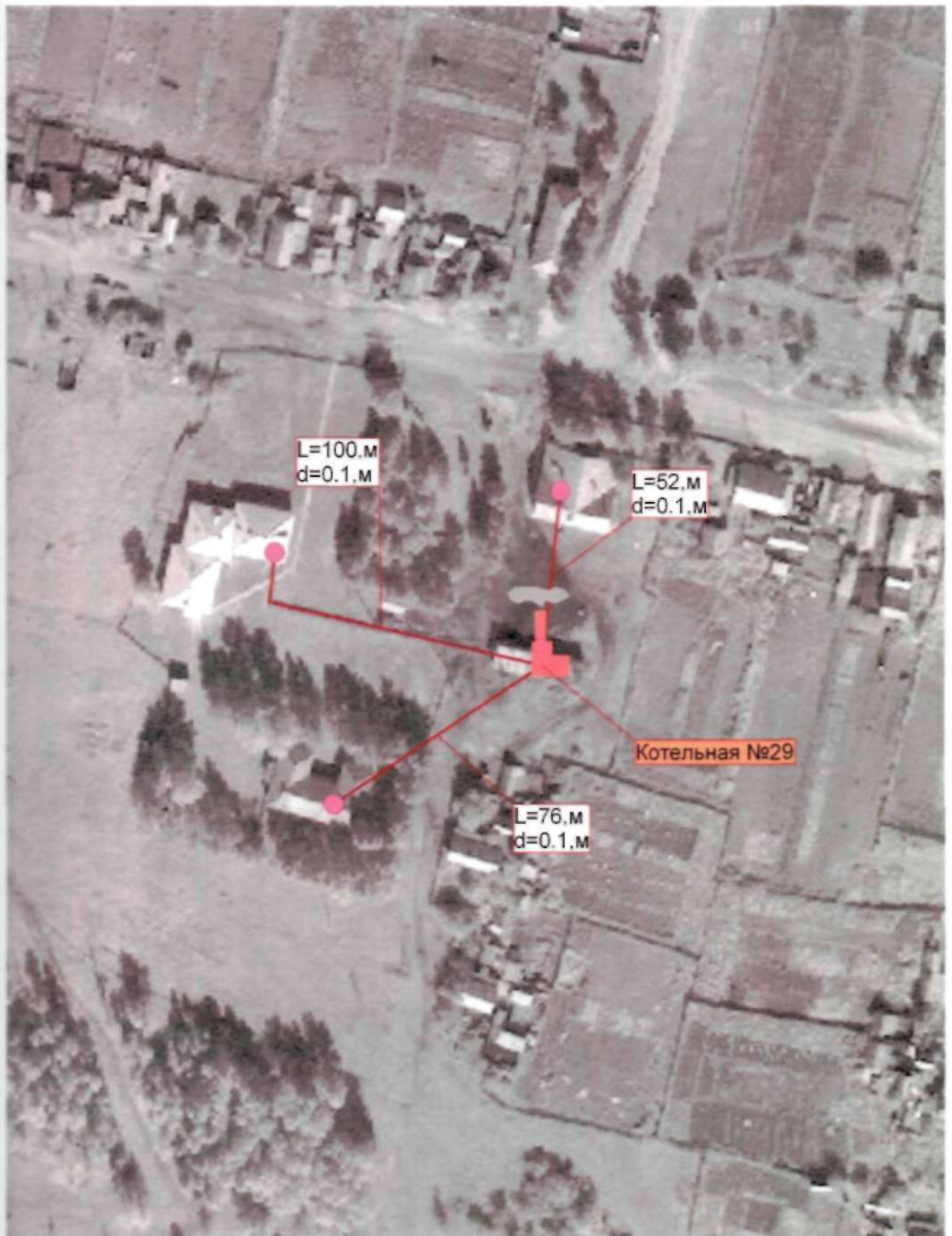
Рис. 2.6 – Схема теплоснабжения муниципального образования "Климоуцевский сельсовет" от котельной №29
